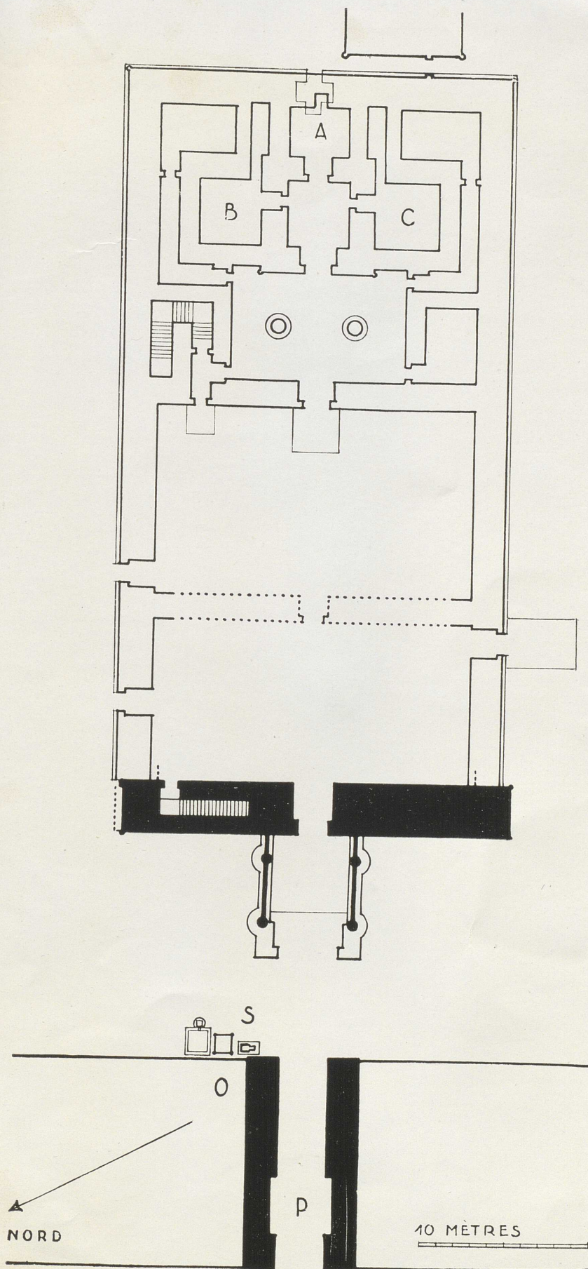
Plan schématique du temple d'Apet.
