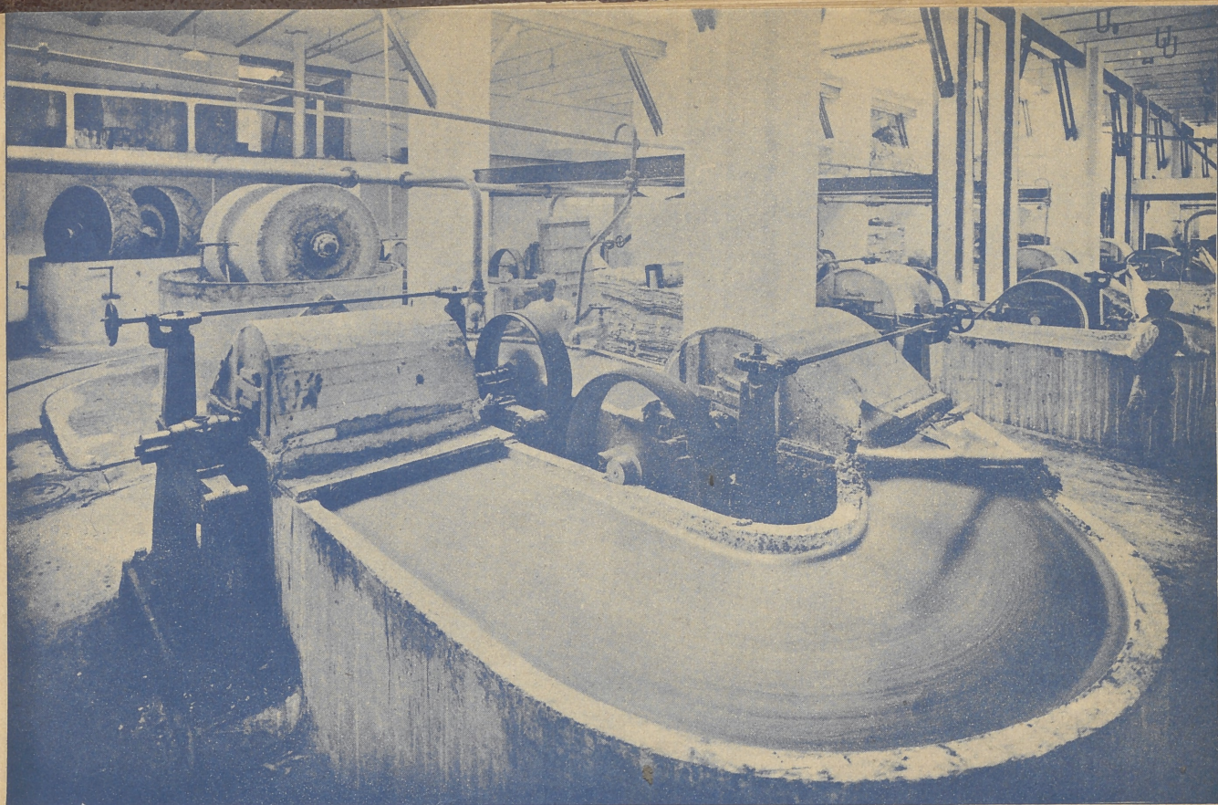
Une "pile" — On voit, derrière, à gauche deux cuves à meules
