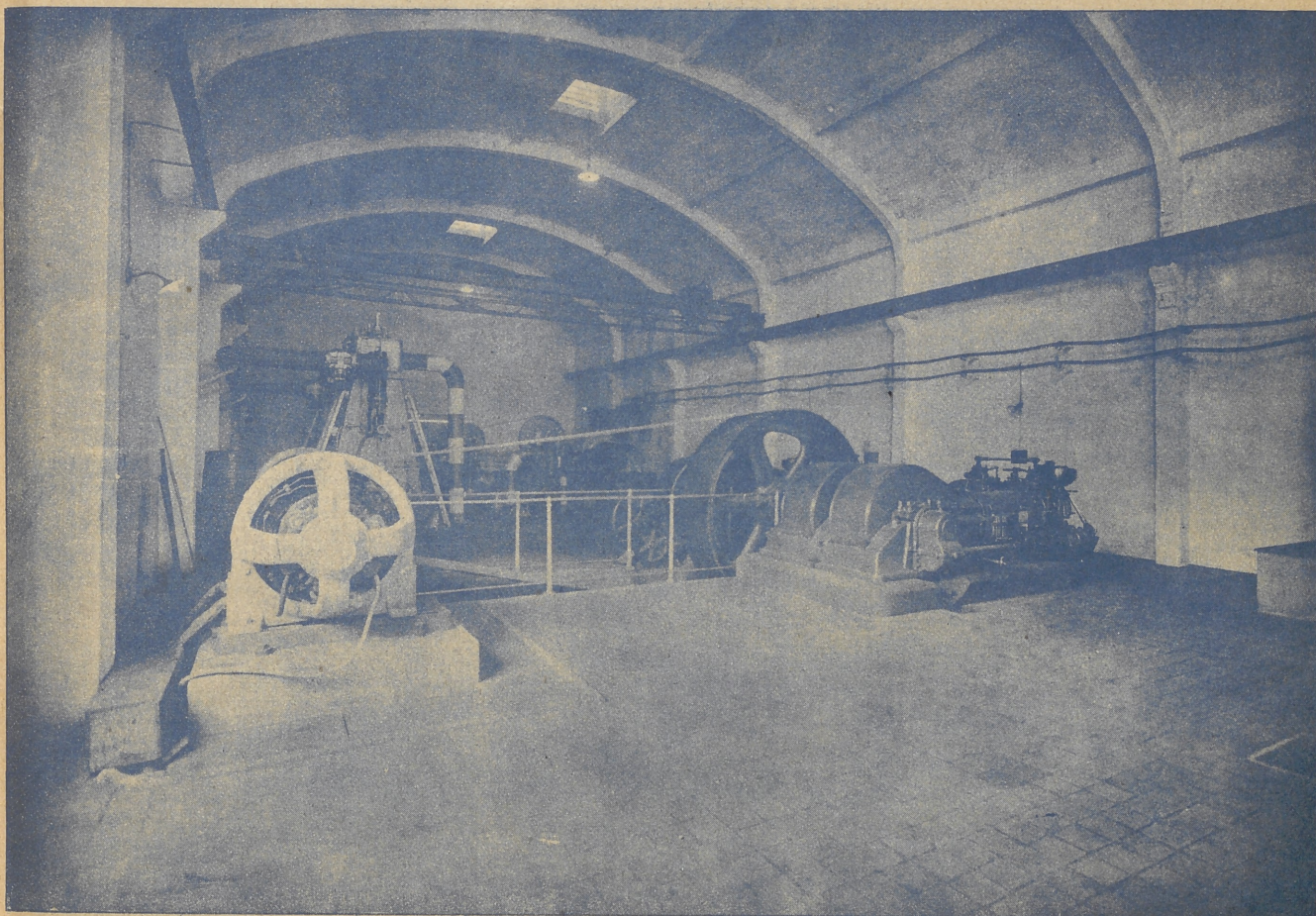
Une partie de la centrale électrique
