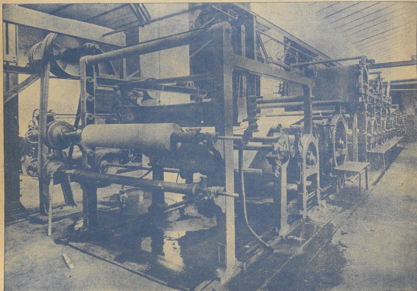
Une machine à papier (c'est la même machine qui s'étend jusqu'au fond de la salle)
