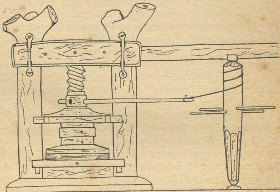
FIG. 121. La presse de Valeyre.
