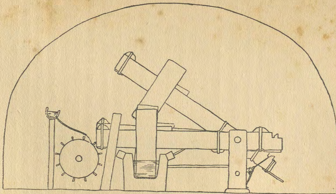
FIG. 119. Détail des marteaux, sous la voûte du moulin.
