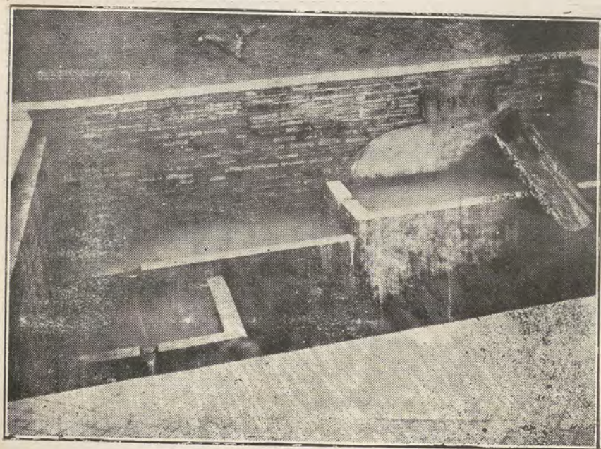
Puits antimalarien du village de XACO 28
