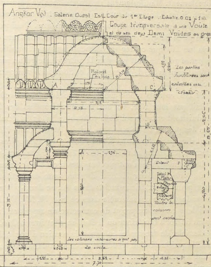
FIG. 111. — Coupe d'une voûte fléchée de deux demi-voûtes : (A. V.).
