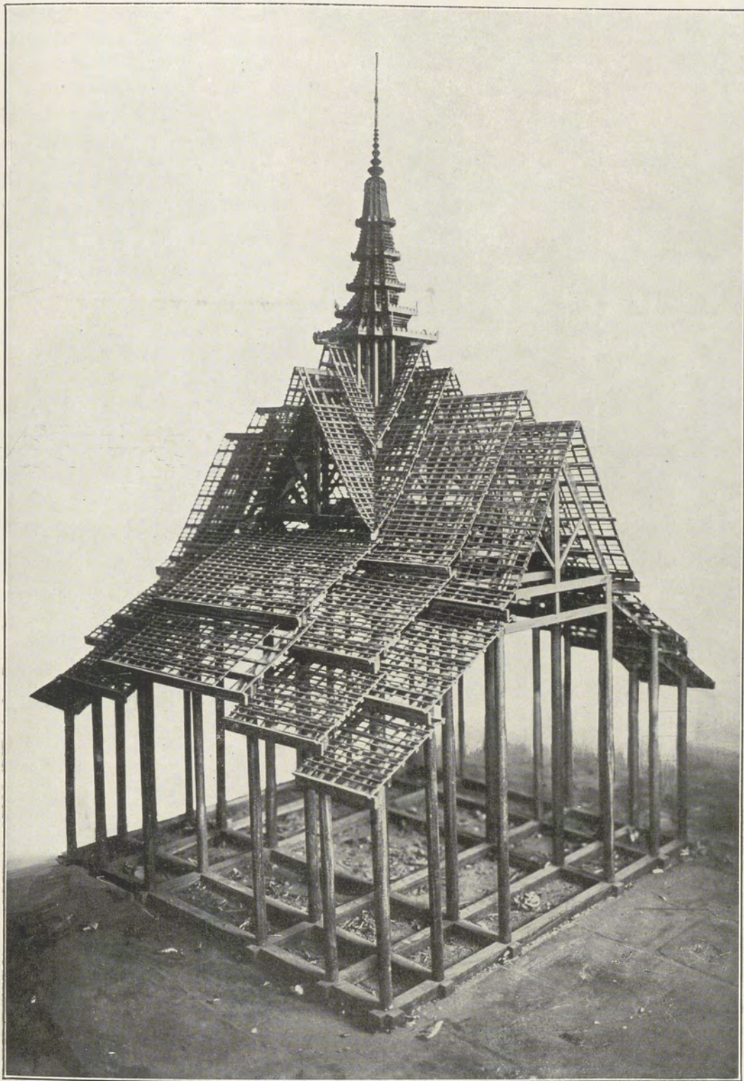
PLANCHE XIX. — Croisée de toitures à double appentis avec décrochements et flèche centrale. Maquette exécutée à l'échelle de 1 pour 10 par l'École des Arts Cambodgiens de Phnom Penh.
