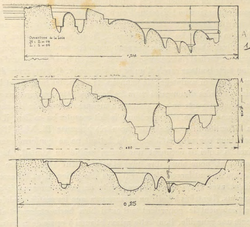
FIG. 145. — Coupes de moulures de cadre de porte.
