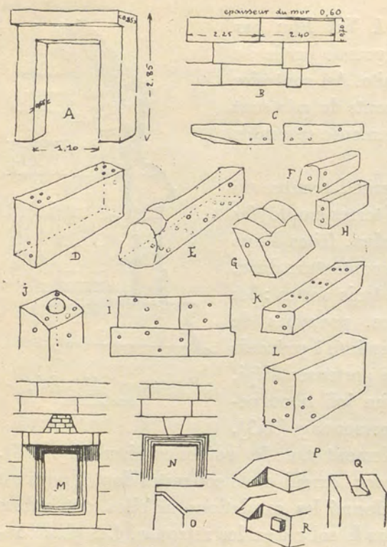
FIG. 103. — Porte monolithe; perforation des pierres; voutins de décharge; assemblages de cadre de porte.
