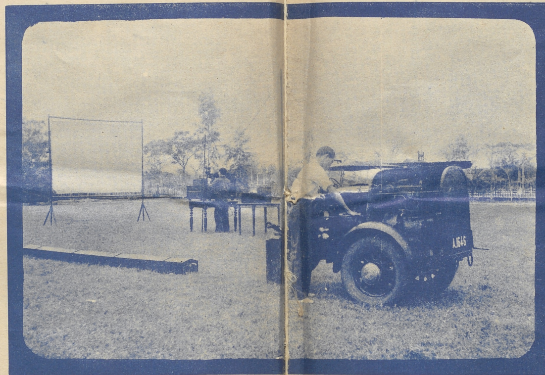
Ensemble du matériel de projection et d'audition monté en plein air (On voit en premier plan le groupe électrogène, en second plan l'appareil de projection, le tourne-disque, le pick-up et le haut-parleur ; dans le fond : l'écran)
