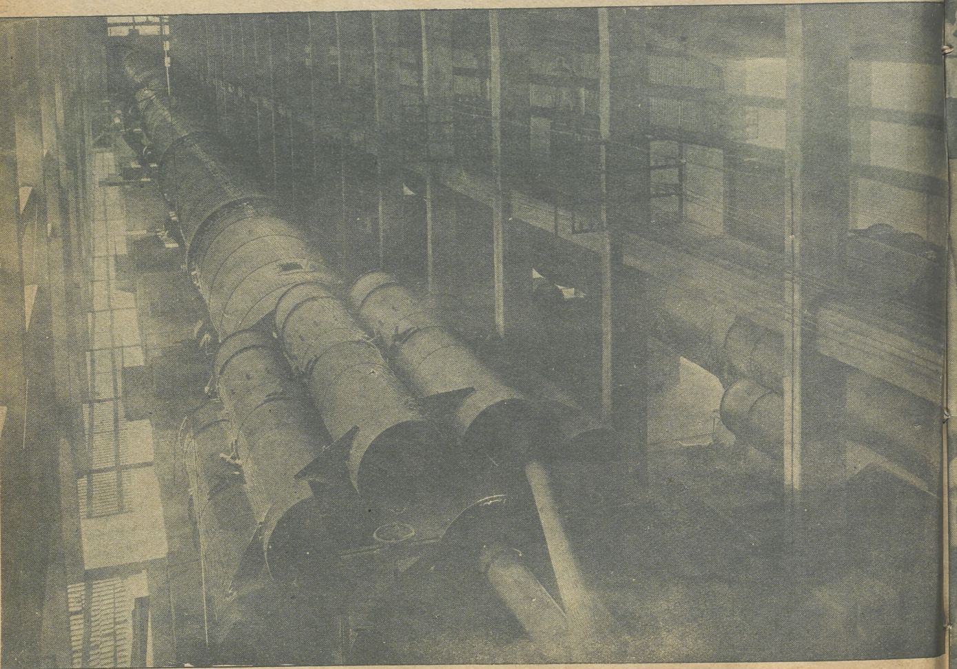
Four à 300 tonnes (longueur 106 m.)
